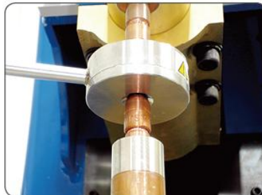
로드셀 하부 사진
